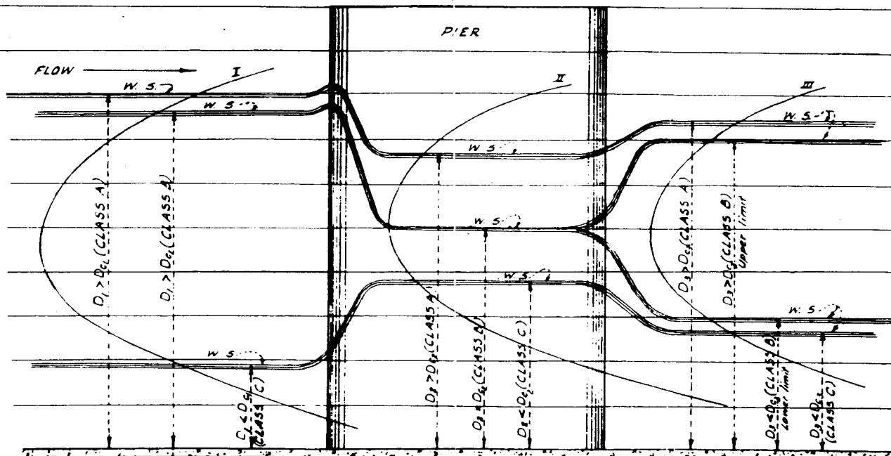
LONGITUDINAL PROFILE
